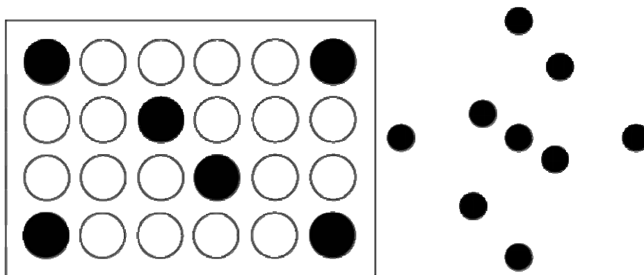
(a) 24孔长方形金属浴模块布点示意图
