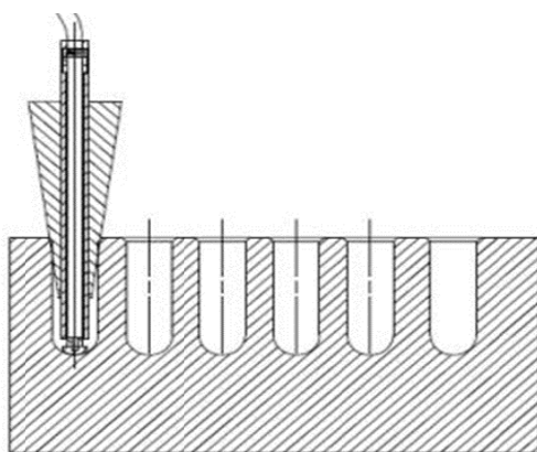
图 1 传感器放置并密封示意图
